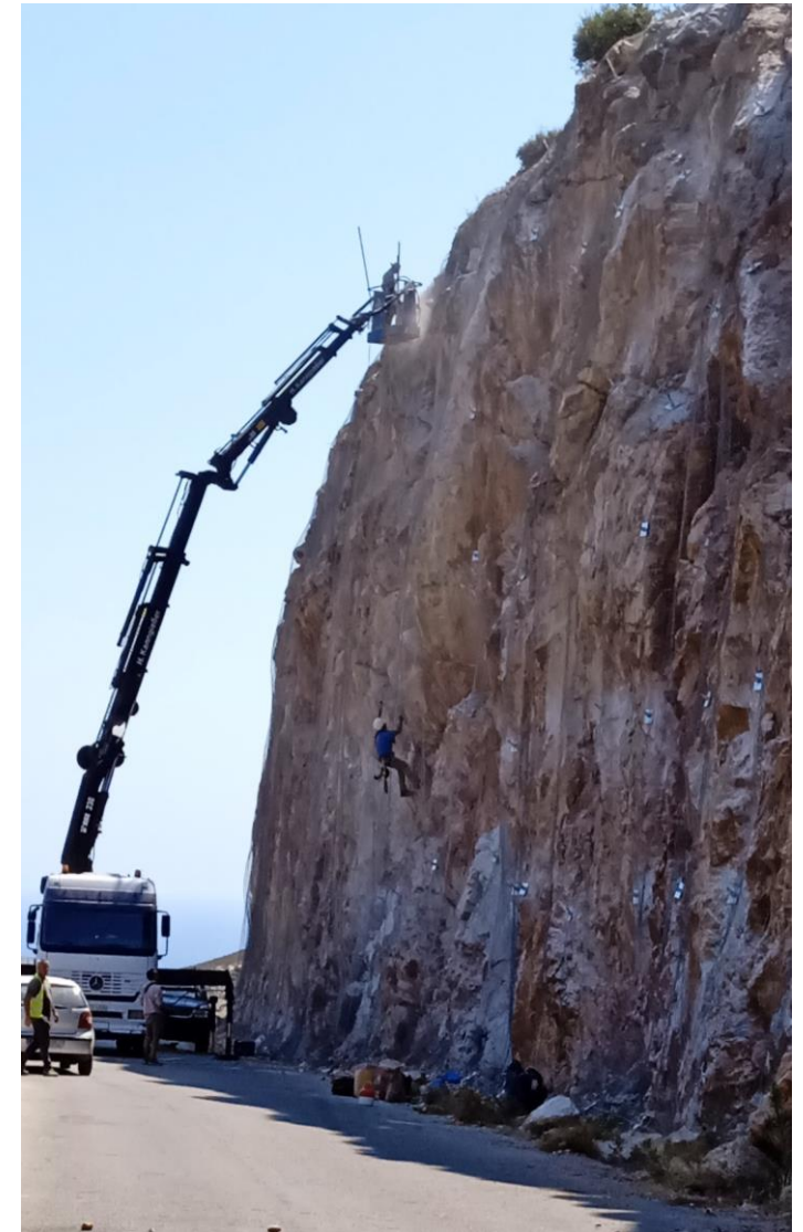
ΕΡΓΑ ΑΝΤΙΜΕΤΩΠΙΣΗΣ ΚΑΤΟΛΙΣΘΗΣΕΩΝ ΣΤΑΥΡΟΣ - ΜΠΑΛΙ
